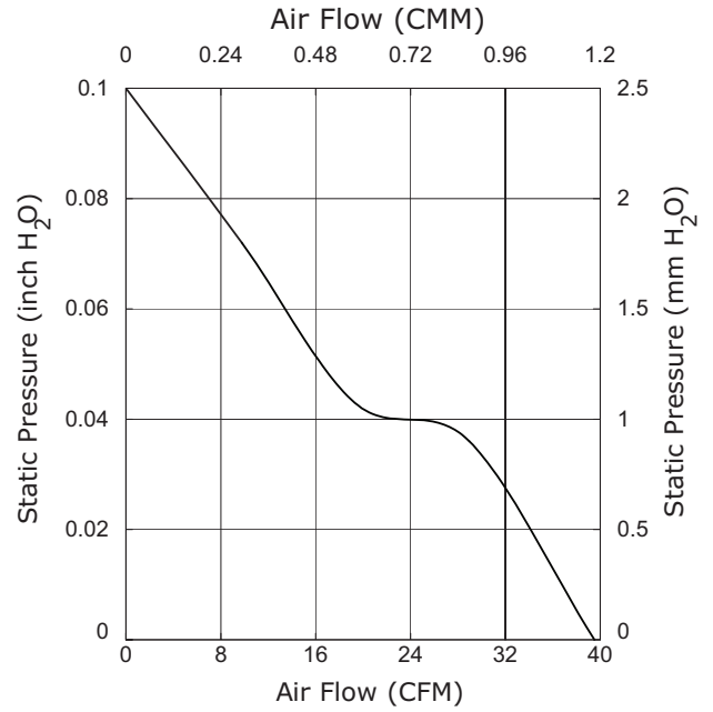
CFM-9225V-130-340
